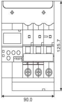
Kích thước sản phẩm (Lắp vừa thanh cài tủ điện)
