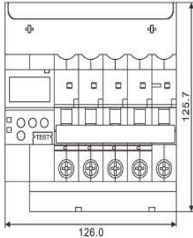
Kích thước sản phẩm (Lắp vừa thanh cài tủ điện)
