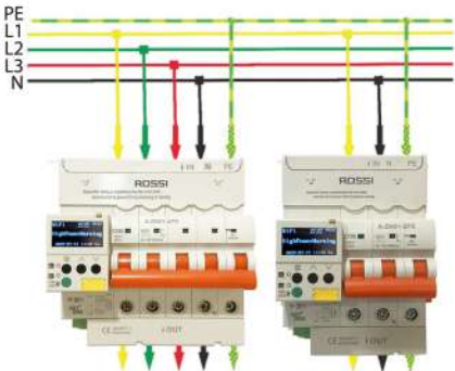
Sơ đồ đấu nối
