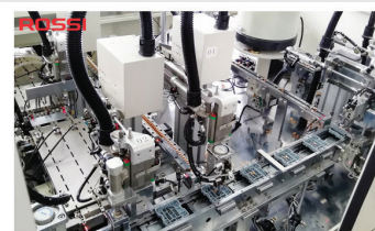
Dây chuyền lắp ráp tự động
